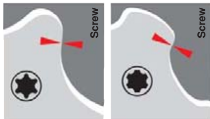
Torx® insert
